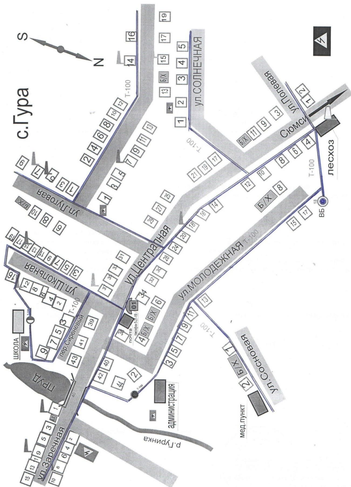
Рисунок 22. Схема водоснабжения с. Гура
