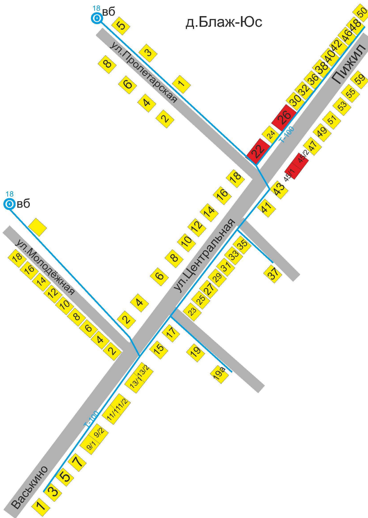
Рисунок 3.Схема водоснабжения д Блаж-Юс
